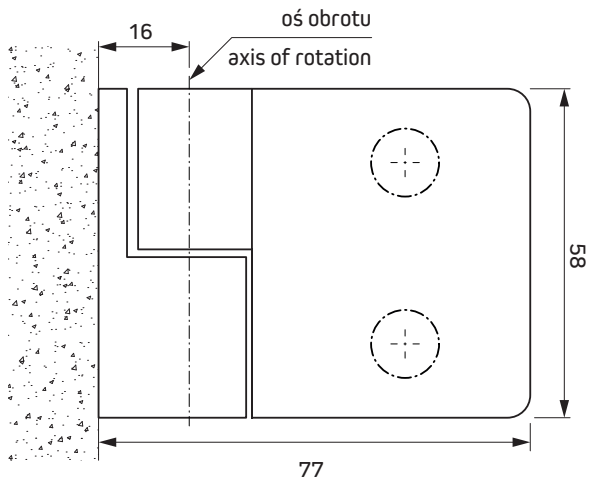
otworowanie zawiasu lewego glass processing for left hinge
