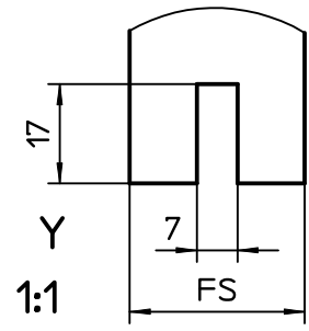
ROLLAN SoftStop Anordnung Trägerplatte / configuration carrier plate
