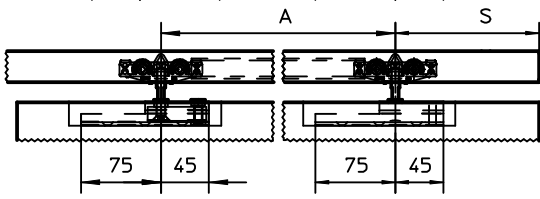
ROLLAN SoftStop Anordnung Trägerplatte / configuration carrier plate
