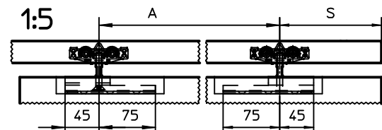
ROLLAN Standard Anordnung Trägerplatte / configuration carrier plate
